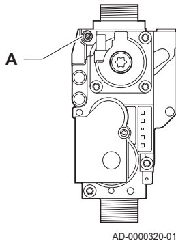
Afb.66 Positie afstelschroef A
