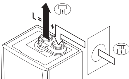
Afb.37 Verschillende drukgebieden
