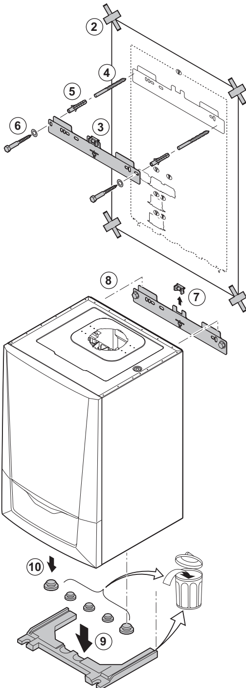
Afb.21 Ophangen ketel
