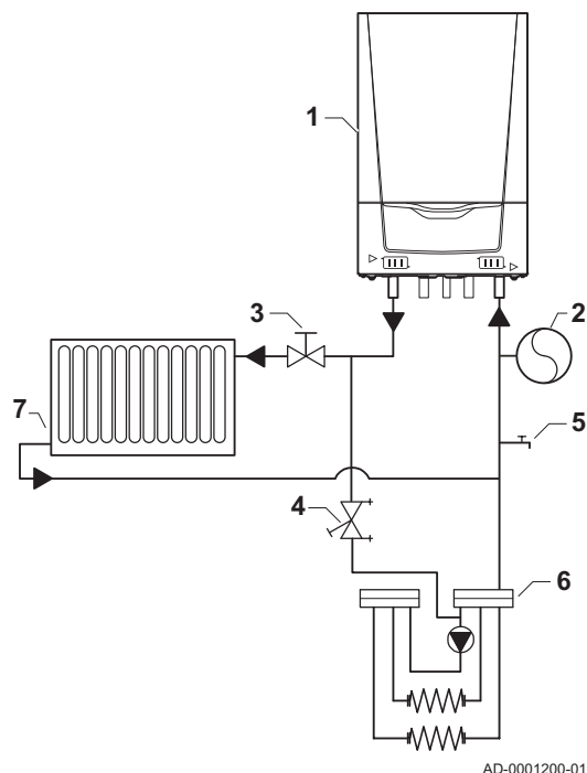
Afb.17 Aansluiting vloerverwarming
