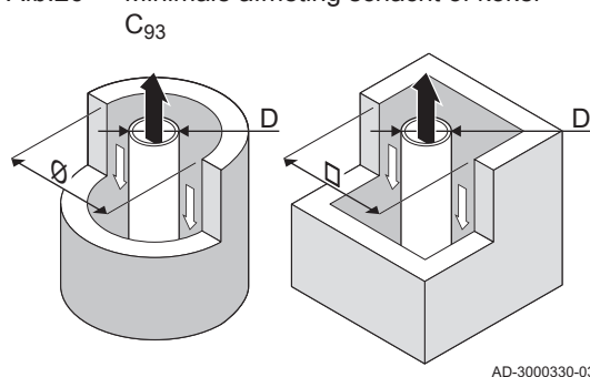
Afb.26 Minimale afmeting schacht of koker
