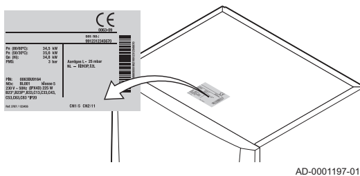
Afb.13 Positie typeplaat
