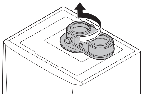
Afb.39 Omdraaien lucht-/rookgasadapter (parallel)
