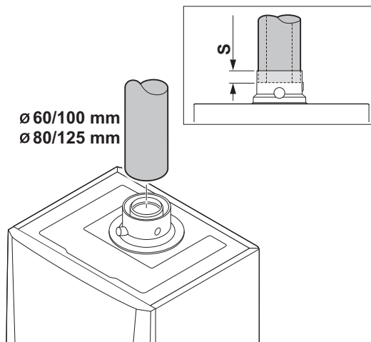
Afb.42 Aansluiten rookgasafvoer en luchttoevoer (concentrisch)
