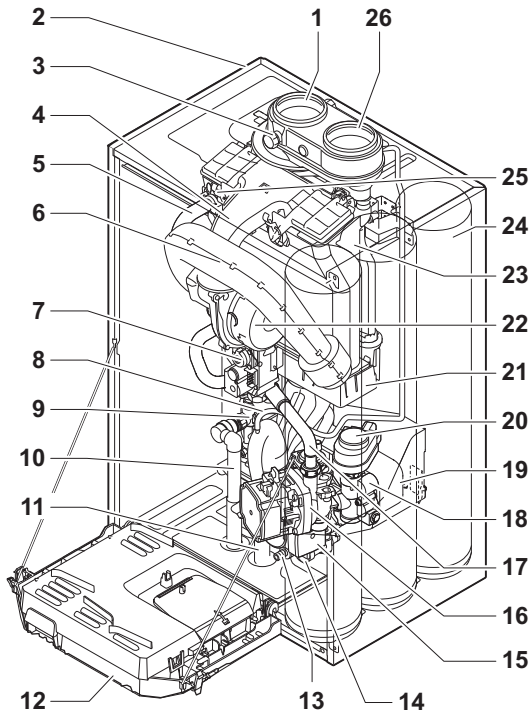
Afb.9 Calenta Ace 40L (parallel)
