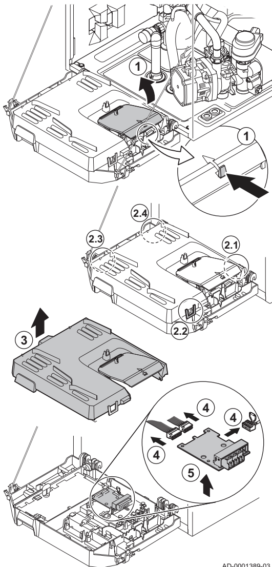
Afb.221 Toegang tot de aansluitconnectoren
