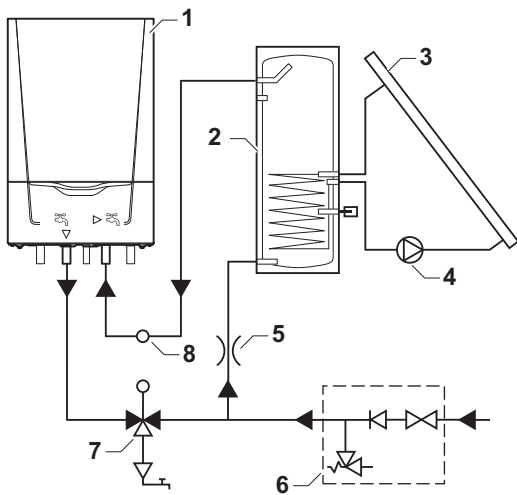
Afb.19 Aansluiten zonneboiler volgens drukgevuuld systeem
