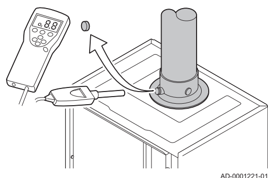
Afb.63 Rookgasmeetpunt
