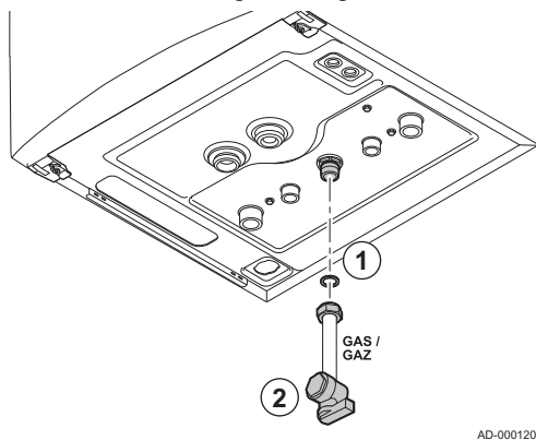
Afb.25 Aansluiten gasleiding
