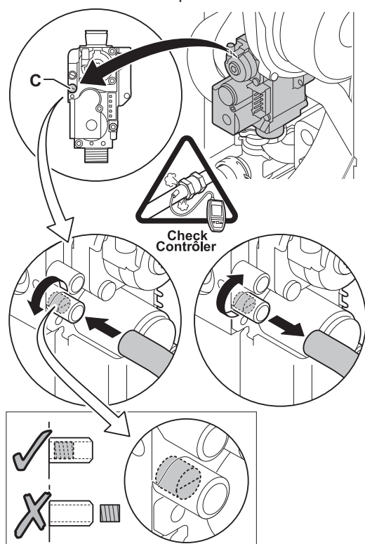
Afb.61 Gasblok meetpunten
