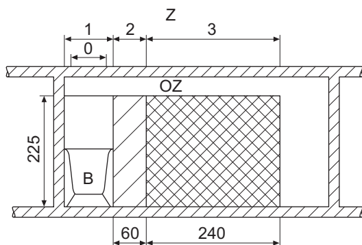
Afb.16 Badkameropstelling
