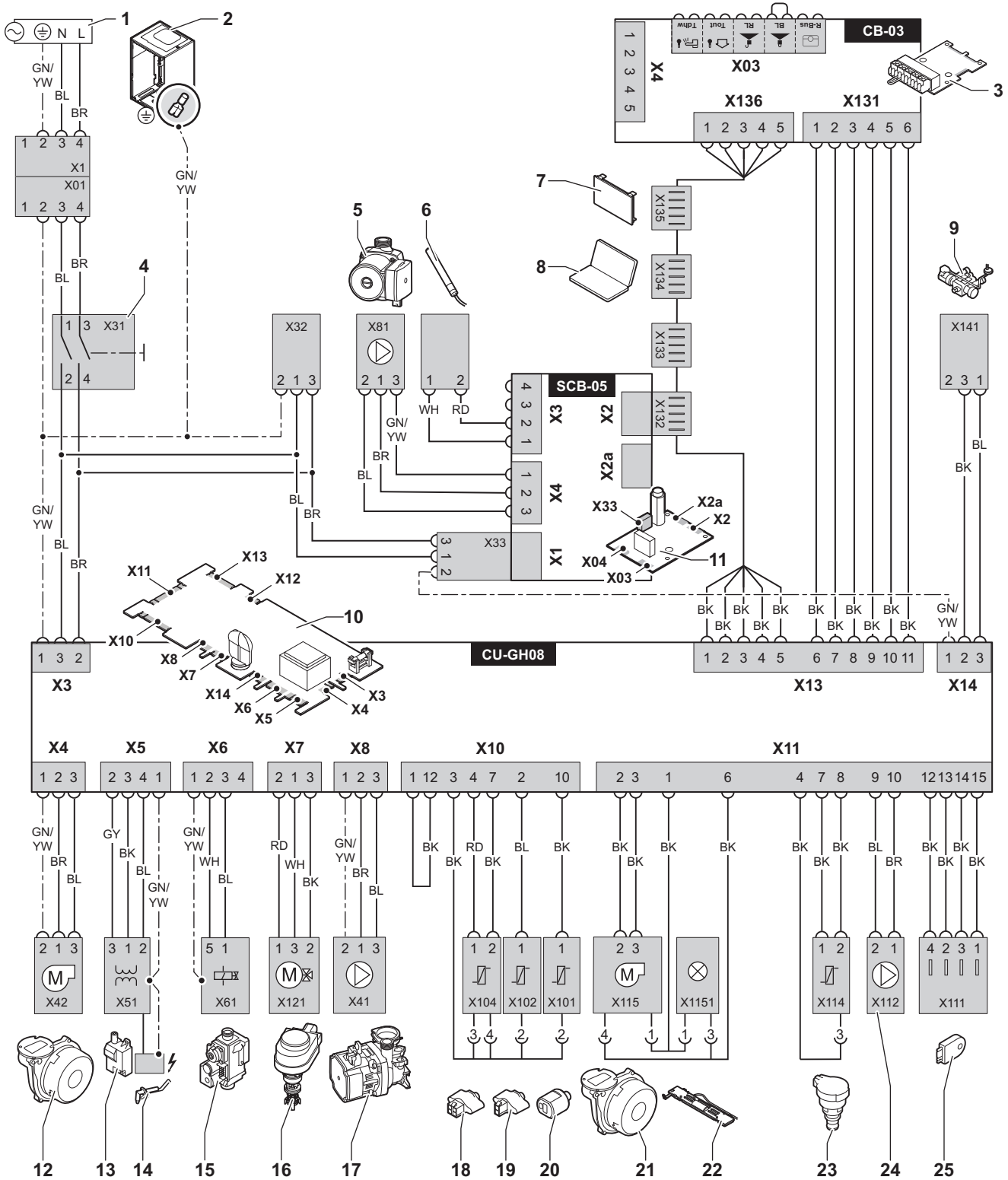
Afb.6 Elektrisch schema
