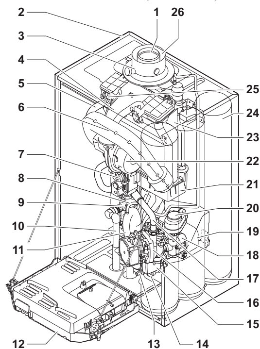
Afb.10 Calenta Ace 40L (concentrisch)
