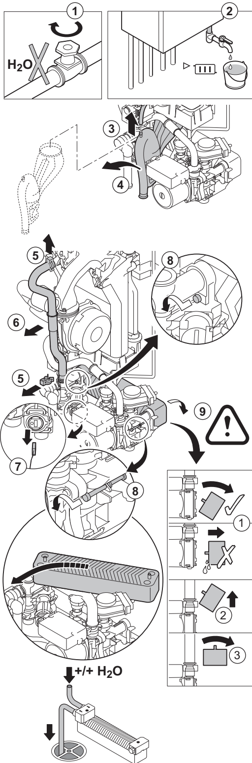
Afb.215 Reiniging platenwarmtewisselaar
