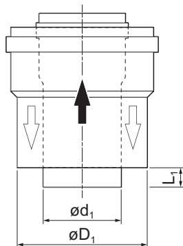
Afb.29 Afmetingen concentrische aansluiting
