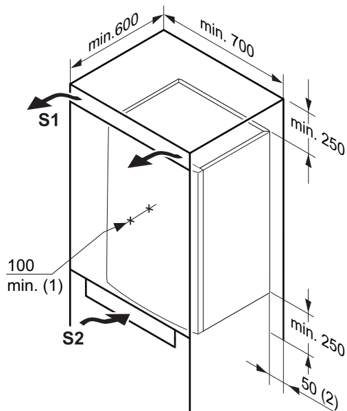
Afb.15 Ruimte voor ventilatie
