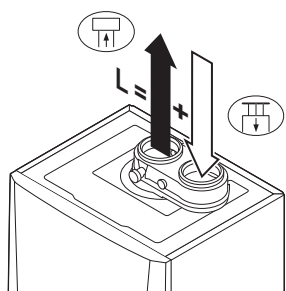
Afb.32 Gesloten uitvoering (parallel)
