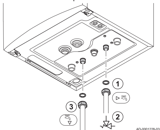
Afb.23 Aansluiten tapwatercircuit
