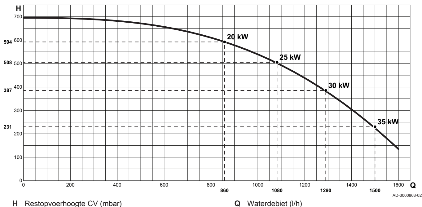
Afb.7 Calenta Ace 40L
