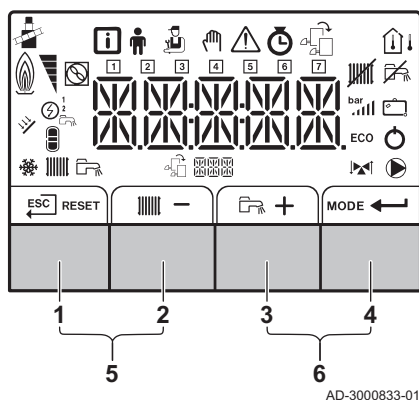
Afb.12 Bedieningspaneel
