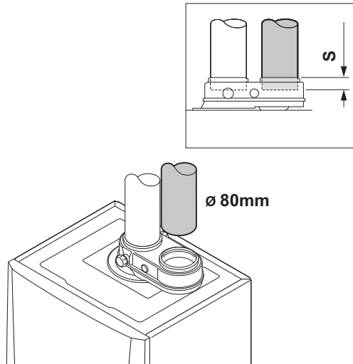
Afb.41 Aansluiten luchttoevoer (parallel)
