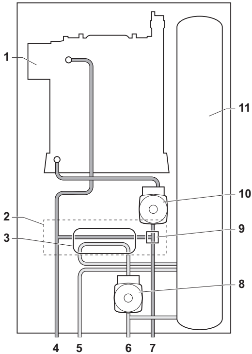
Afb.8 Calenta Ace 40L
