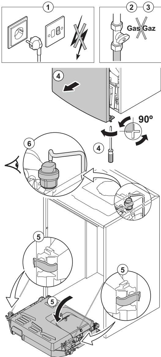
Afb.210 Controle van de automatische ontluucher
