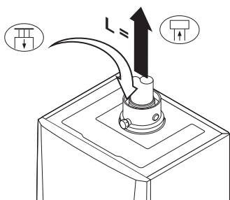
Afb.31 Open uitvoering (concentrisch)
