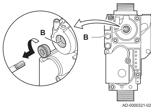
Afb.68 Positie afstelschroef B
