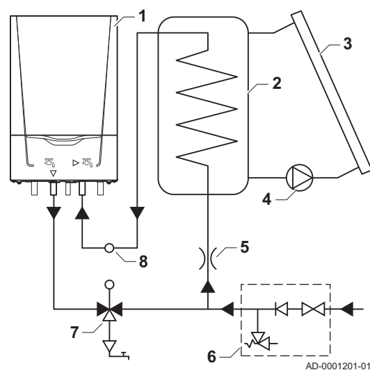
Afb.18 Aansluiten zonneboiler volgens terugloopsysteem
