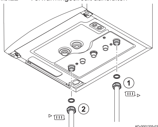
Afb.22 Verwarmingscircuit aansluiten
