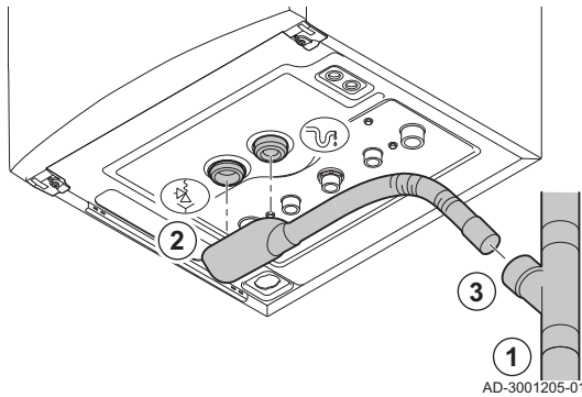
Afb.24 Condensafvoerbuis aansluiten
