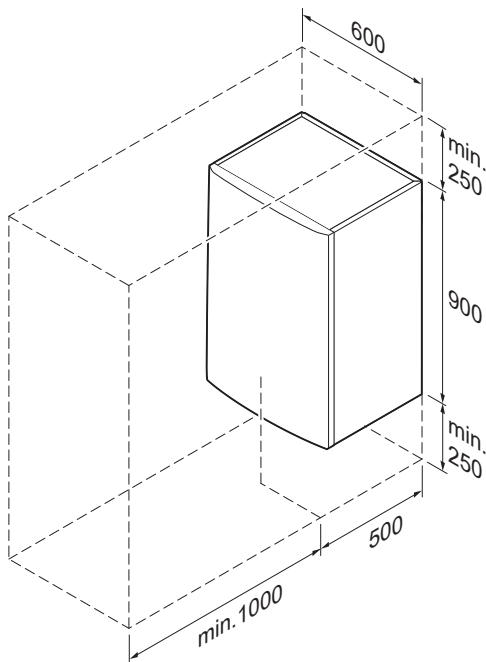
Afb.14 Montageruimte
