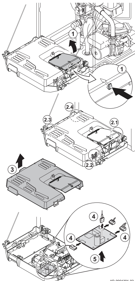
Afb.222 Toegang tot de aansluitconnectoren
