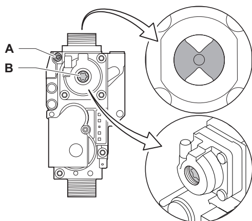
Afb.69 Gasblok
