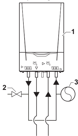
Afb.20 Geiser-toepassing
