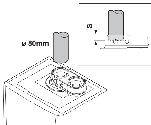
Afb.40 Aansluiten rookgasafvoer (parallel)
