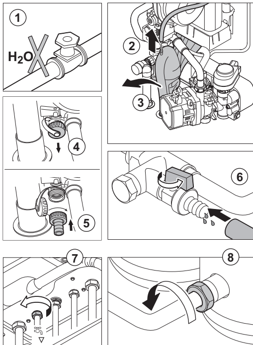
Afb.217 Vervangen boilervaten
