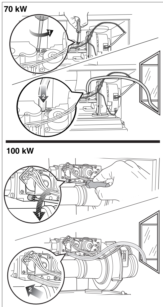
Fig. 67 Gastoevoerleiding ontlichten
