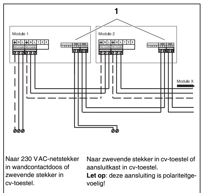
Fig. 44 Meerdere modules
