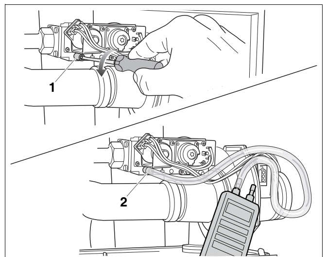
Fig. 90 Gasaansluitdruk meten
