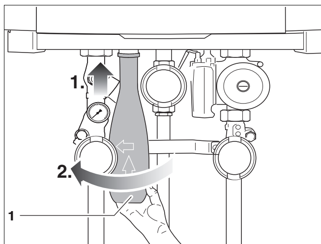
Fig. 17 Toestelsifon monteren
