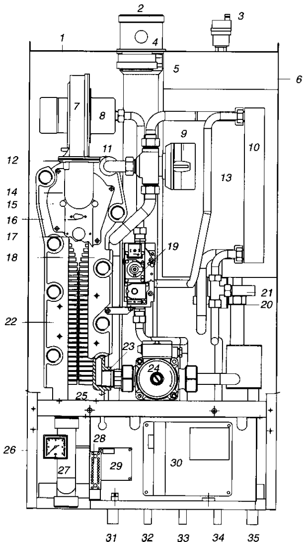
Afb. 06 Doorsnede remeha W21/28c ECO
