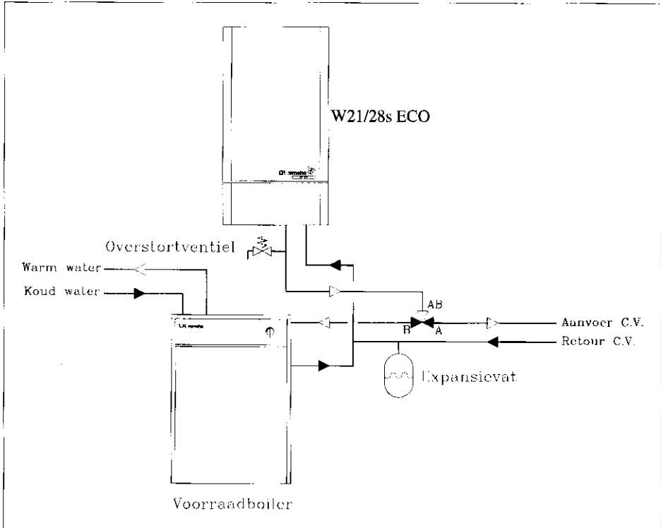
Afb. 14 Principeschema W21/28s ECO met voorraadboiler
