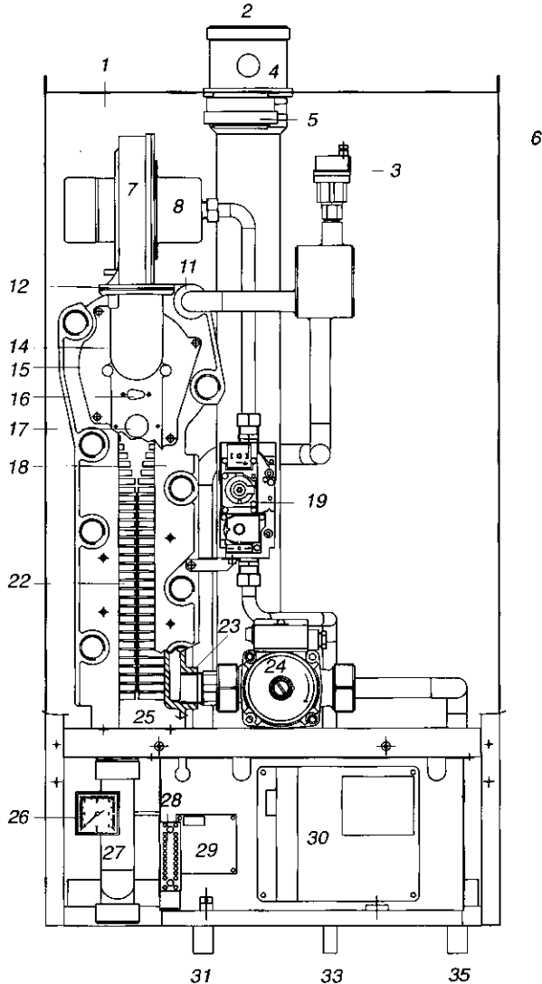
Afb. 05 Doorsnede remeha W21/28s ECO
