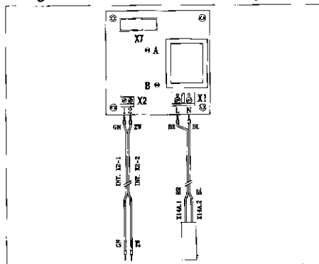
Afb. 20 Interfaceprint t.b.v. modulerende ruimteregelaar
