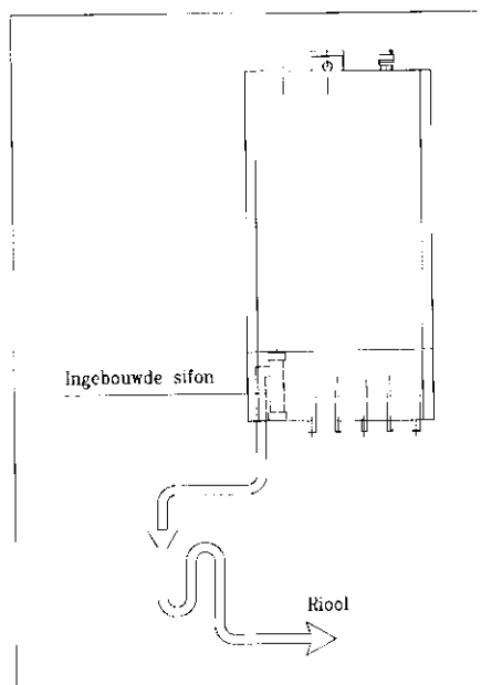
Afb. 11 Condensafvoer
