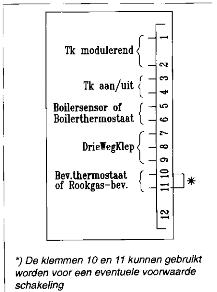
Afb. 15 Aansluitingen op klemmenstrook
