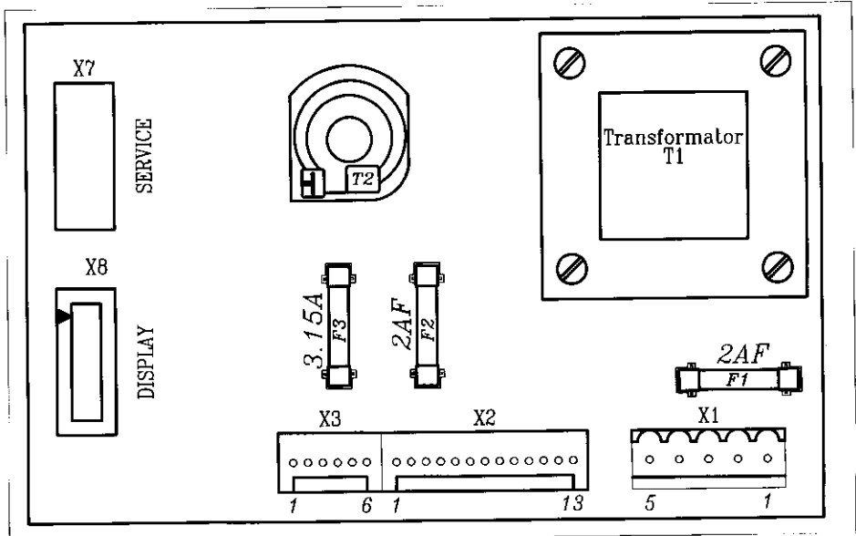
Afb. 16 Beveiligingsautomaat Gasmodul
