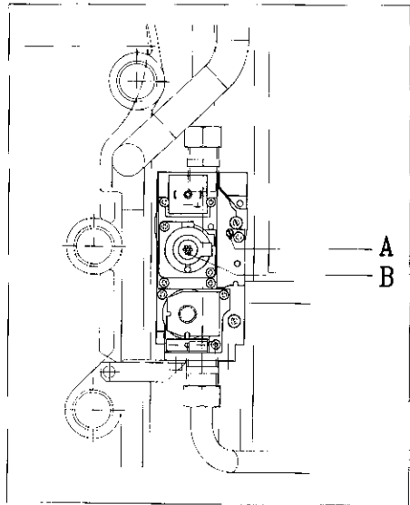
Afb. 19 Instelpunten
