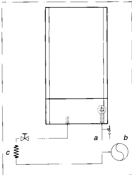
Afb. 13 Veiligheidsvoorzieningen
