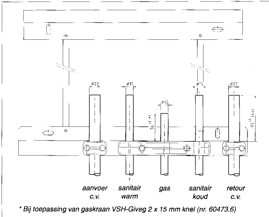
Afb. 10 Montagebeugel (optie)
