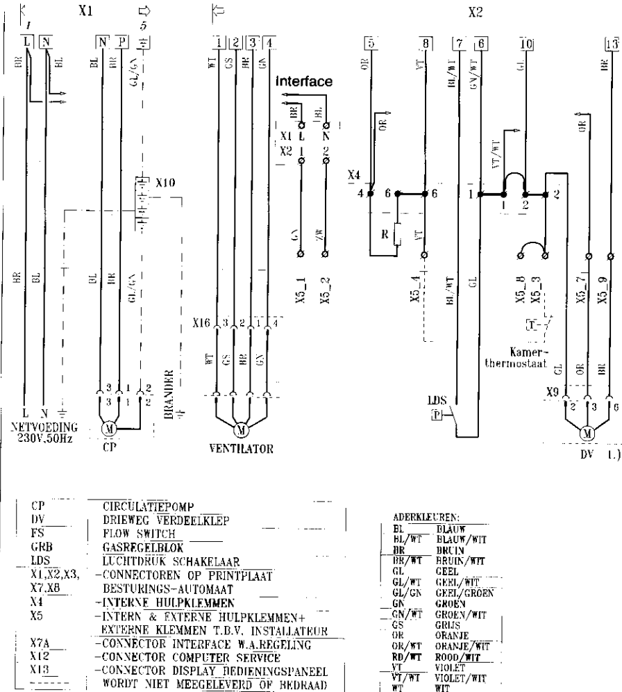
Afb. 17a Elektrisch schema deel 1
