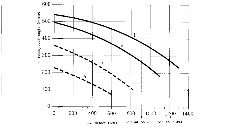
Afb. 12 Grafiek restopvoerhoogte t.b.v. de c.v.-installatie
