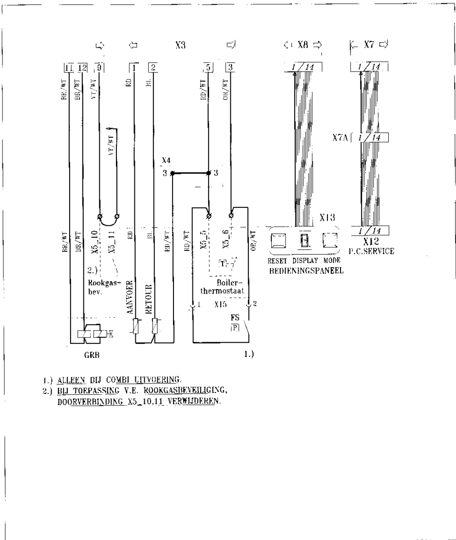
Afb. 17b Elektrisch schema deel 2
