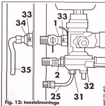
Fig. 12: toestelmontage
