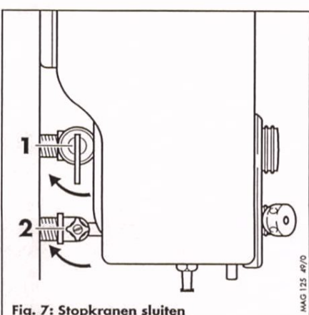
Fig. 7: Stopkranen sluiten
