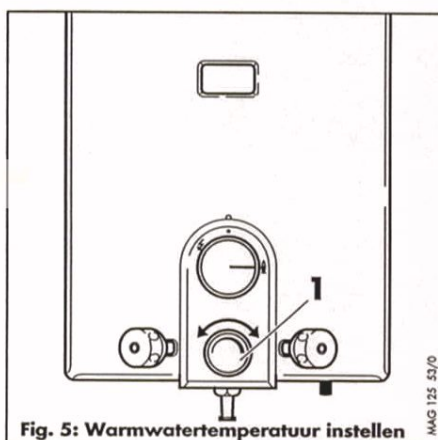
Fig. 5: Warmwatertemperatuur instellen
