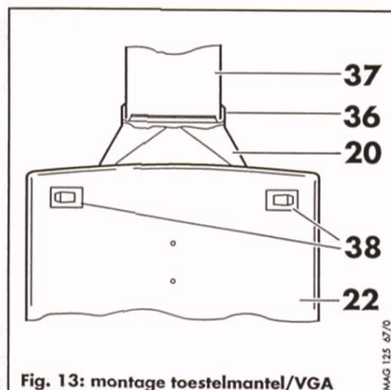
Fig. 13: montage toestelmantel/VGA
